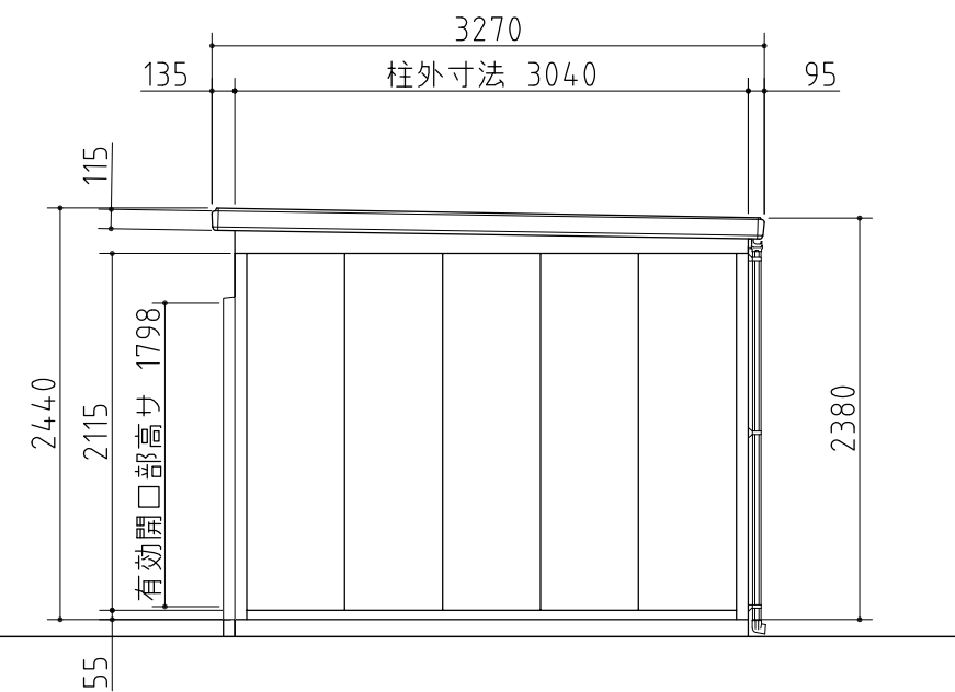
右側面図
