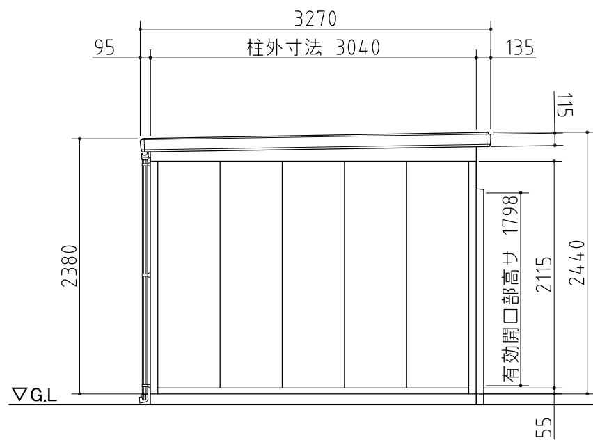
左側面図
